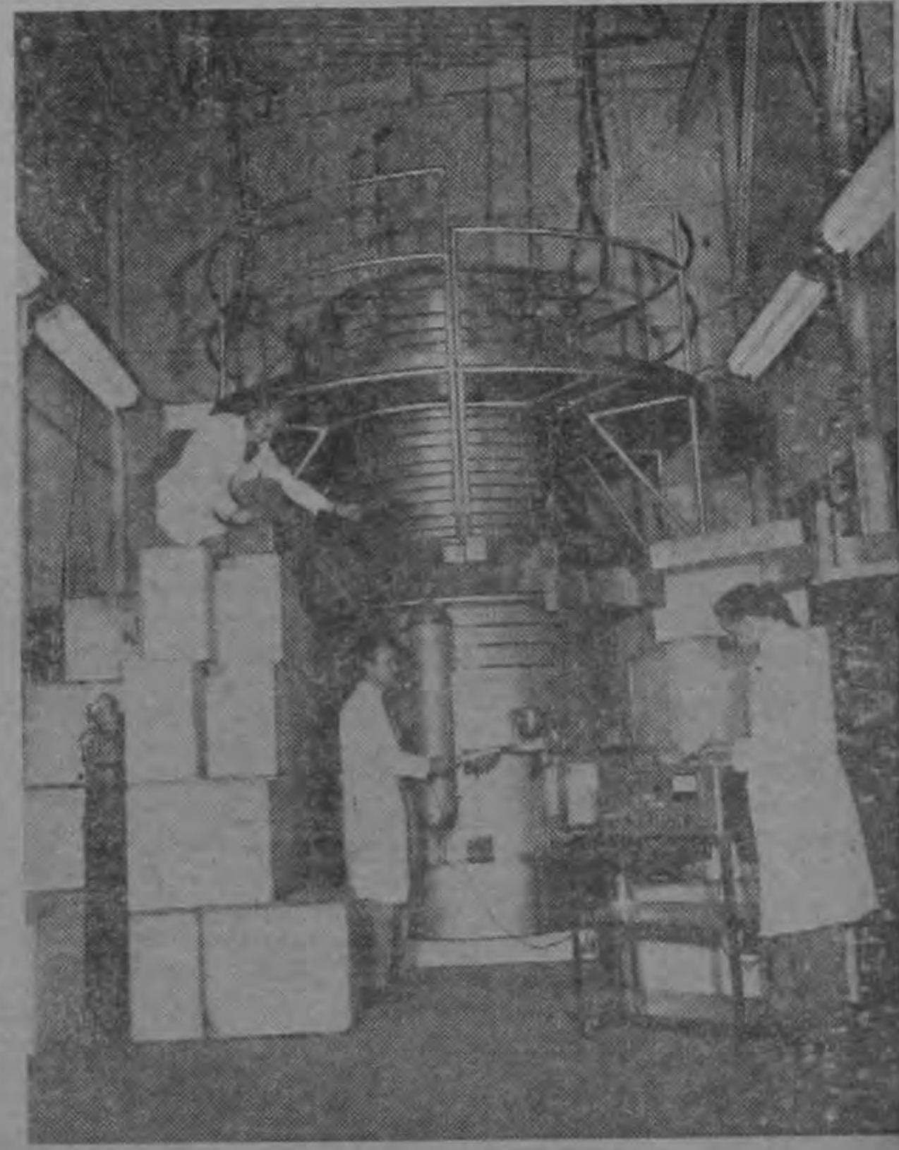
En ocasión de estarse celebrando la importante Conferencia para usos pacíficos de la energía atómica en Ginebra, es oportuno dar a conocer a nuestros lectores el reactor atómico que figura en la fotografía. Es un reactor del tipo llamado hervidores de agua, construido por la compañía "North American Aviation". Para tomar esta foto se corrieron algunos de los gruesos bloques de concreto que normalmente sirven de protección, para dejar ver el reactor. Los técnicos están midiendo, con contadores Geiger, cualquier pequeña cantidad de radiación que se haya escapado. (Foto USIS).
